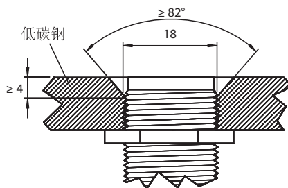
接近开关感应面与安装面齐平。
